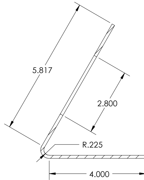
SECTION A-A SCALE 1 : 2
